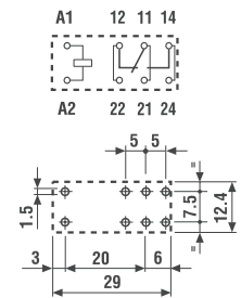
Ansicht auf die Anschlüsse
