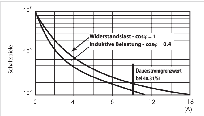
F 40.5 - Elektrische Lebensdauer bei AC
