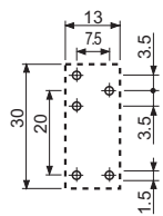
Ansicht auf die Anschlüsse
