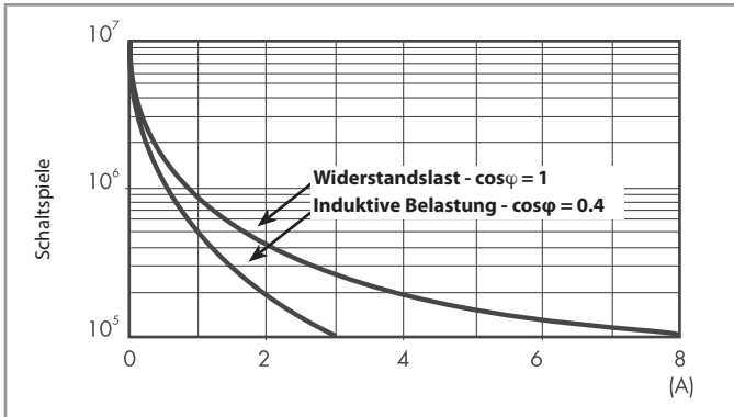
F 40.4 - Elektrische Lebensdauer bei AC
