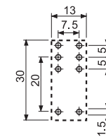
Ansicht auf die Anschlüsse
