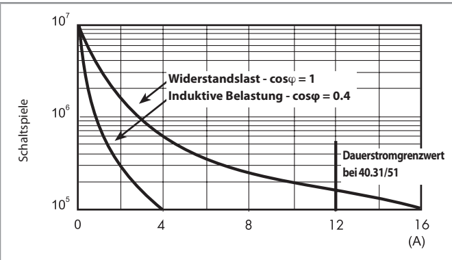
F 40.3 - Elektrische Lebensdauer bei AC
