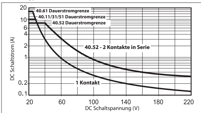
H 40.2 - Gleichstromschaltvermögen bei DC1 - Belastung
