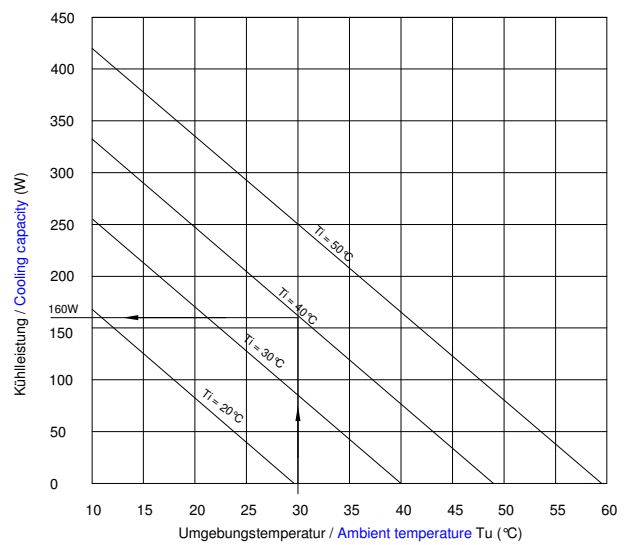
Leistungsdiagramm / Performance curve PK 75
